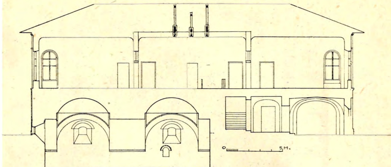
Fig. 7. — Secția Nord-Sud
