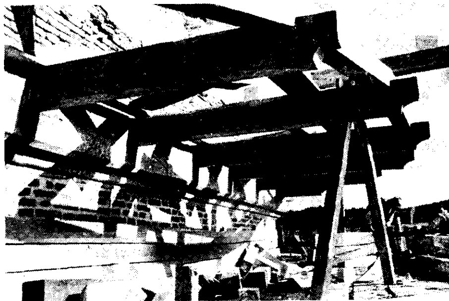
Fig.6. Noua Streasină a bisericii. Console de pe latura de vest în timpul lucrărilor de refacere a acoperișului.
