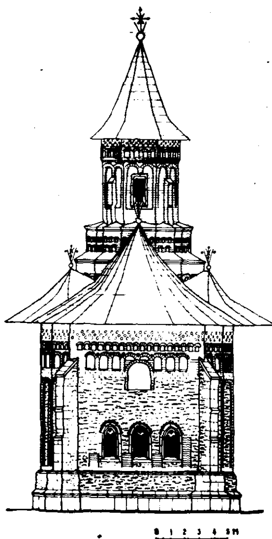
Fig.11. Biserica lui Stefan cel Mare. Fațada de vest după restaurare. Elevație.
