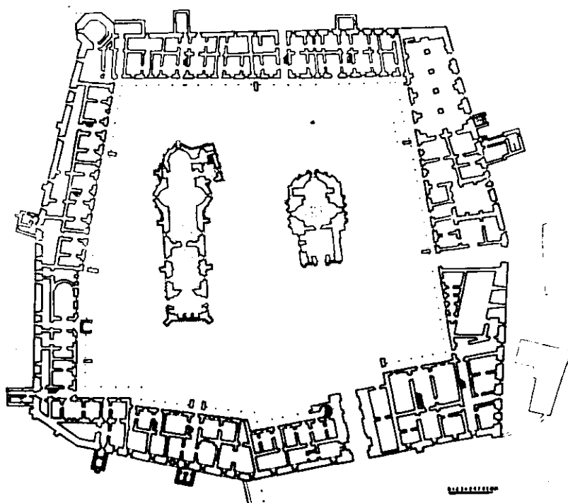
Fig.15. Planul incintei, parter, înainte de restaurare.
