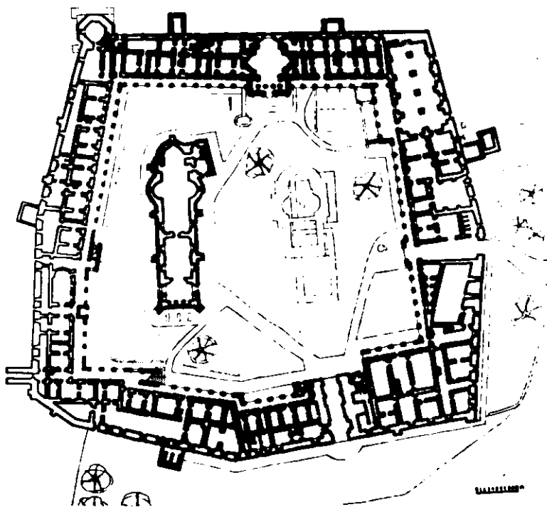
Fig.16. Planul incintei după restaurare.
