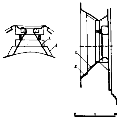
Fig. 7. Detaliu de fereastră la absida de sud. Plan și secție. 1) Golul restaurat. 2) Golul ferestrei din secolul al XIX-lea.
