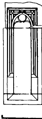
Fig. 8. Chenar de fereastră reconstituit la gropniță.
