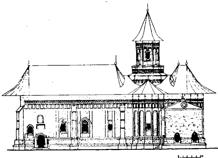
Fig.10. Biserica lui Stefan cel Mare. Fațada de sud după restaurare. Elevație.
