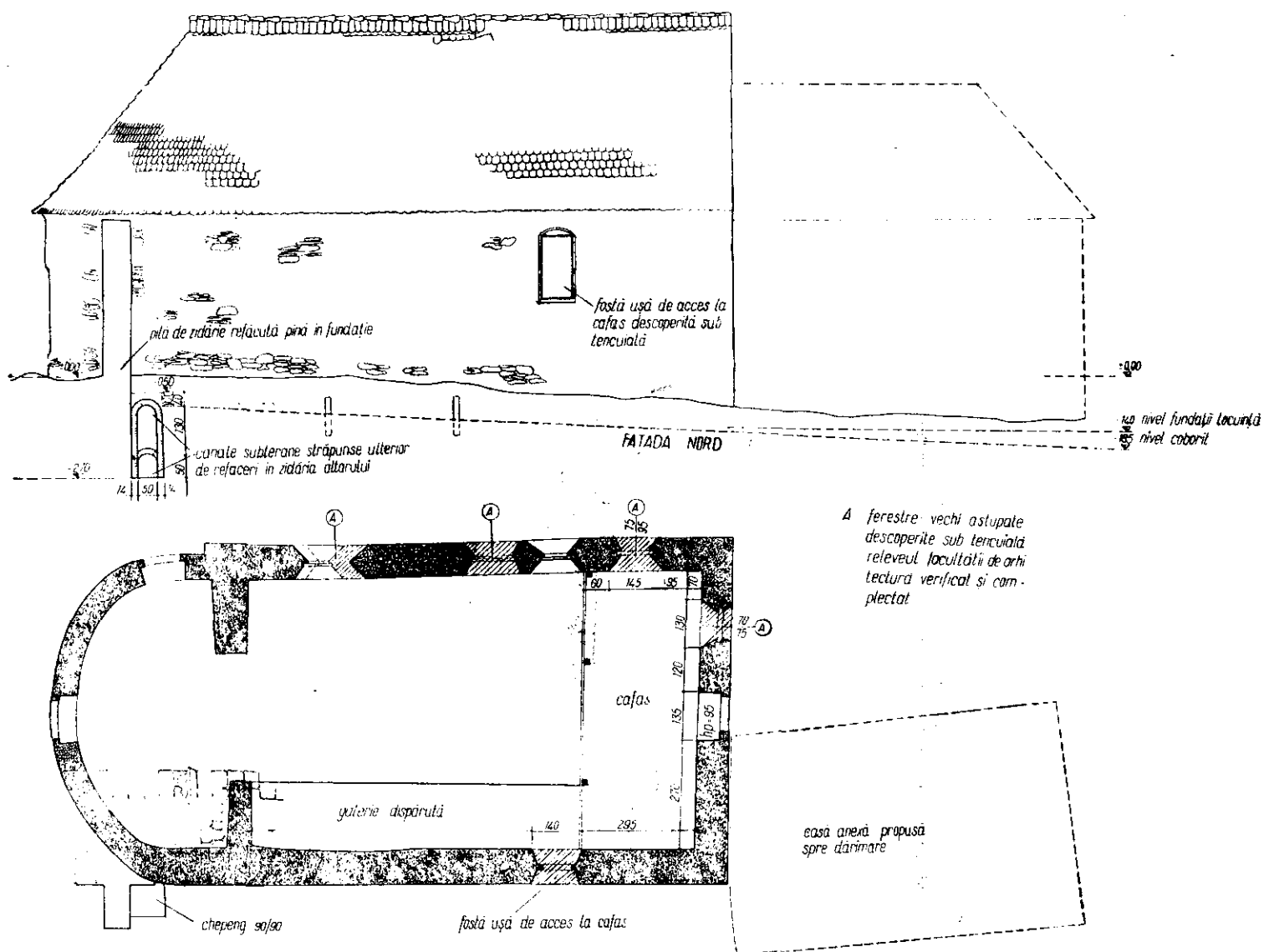
11 a. Capela. Fațadă nord, plan.
