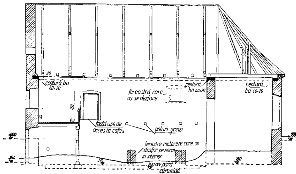
11 b. Capela. Secțiuni longitudinale. 11 b. Coupes longitudinales de la chapelle.
