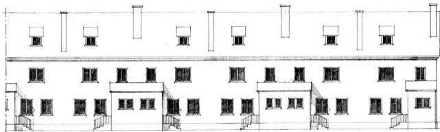
FAJADA SPRE CURTE.
