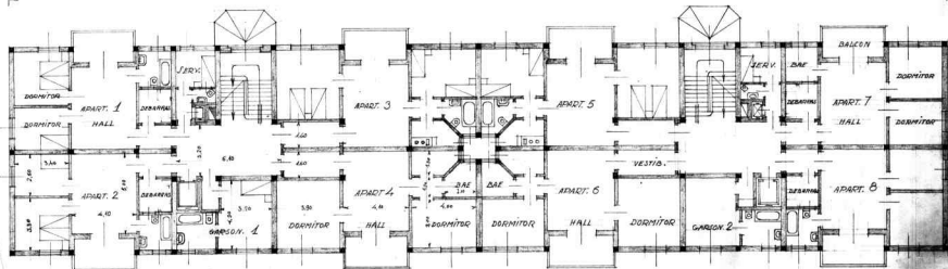
PLANUL ETAJELOR II-III
