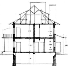
SECȚIE A-B.
