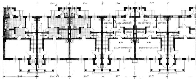
PLANUL PARTERULUI
