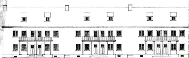
FAȚADA SPRE STRADĂ
