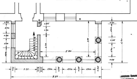
PLAN ETAJ
