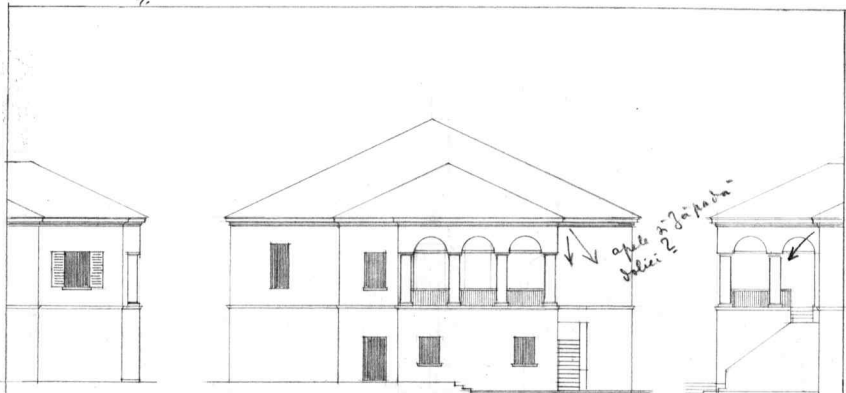
PALATUL EPISCOPAL HUȘI PROECT PENTRU TRANSF. FAȚADEI SUD. SCARA 1CM. — MAI 1936. — ARHITECT Dr. D. J.
