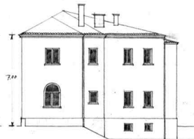
FATADA LATERALĂ
