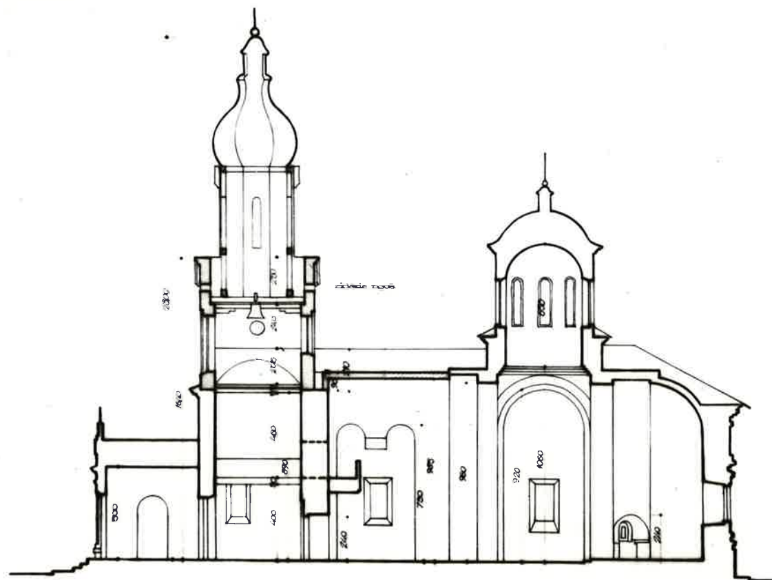
secțiune longitudinală - relevu -
