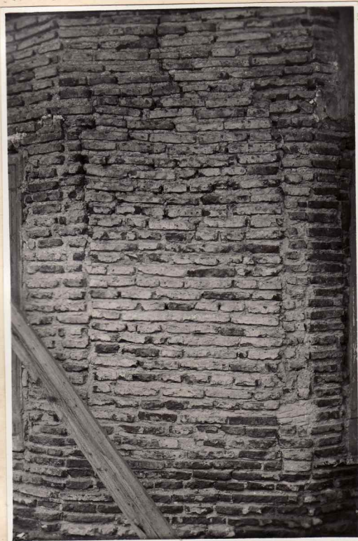
1. Absida laterală sud. Se observă urma vechii ferestre din axul absidei care a fost astupată, deschizându-se cele 2 actuale care se observă în dreapta și stînga (cadru de piatră)
