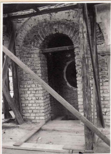
1. Arcada stîngă de pe fațada vest micșorată cu cărămidă modernă. Arcada era mai mare (vezi arcul deasupra). Pentru a se sprijini arcul s-a tăiat zidăria deasupra capitelului (vezi în dreapta).
