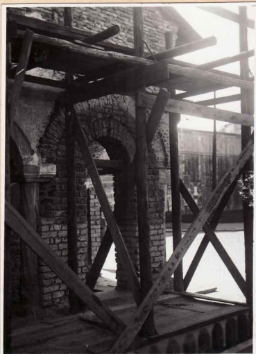
2. Colțul sud-vest. Se observă cele 2 perioade de schimbări. I. Adăugirea părții laterale tăindu-se zidăria peste capitel pentru sprijinirea arcului. II. Umplătura cu cărămidă modernă pentru micșorarea golului.
